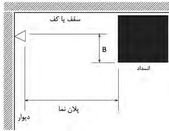
شکل ۴-۶-۱۰- موقعیت اسپرینکلرهای دیواری تا مانع
