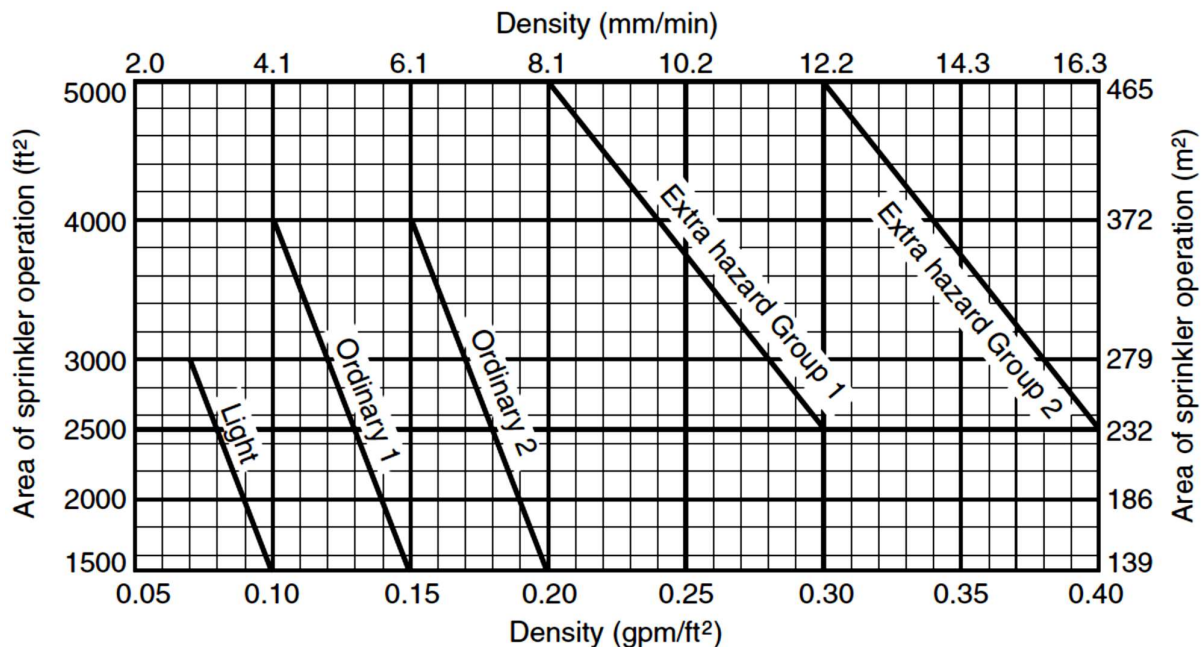
نمودار ۴-۷-۶- منحنی چگالی / مساحت
