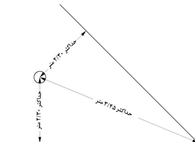
شکل ۴-۴-۱۱- حداکثر فاصله اسپرینکلر از کنج دیوار
